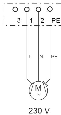
Fig. 364: MS2N Fan connection 230 V
