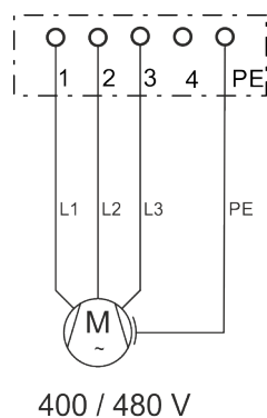
Fig. 365: MS2N Fan connection 400 / 480 V
