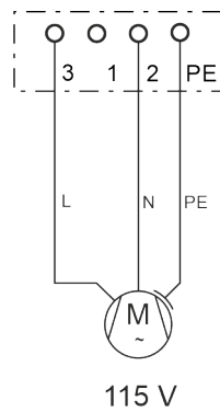
Fig. 363: MS2N Fan connection 115 V
